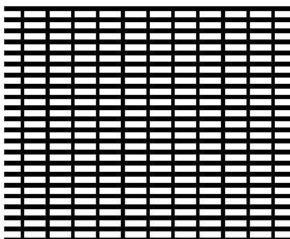
Nr. 4086 mm Lochweite b x h 4,0 x 1,1 Teilung horizontal 4,8 Teilung vertikal 2,1 Durchlass 44 %
