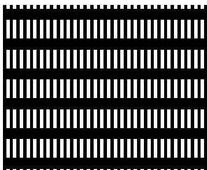
Nr. 4120 mm Lochweite b x h 0,8 x 5,0 Teilung horizontal 1,8 Teilung vertikal 8,0 Durchlass 28 %
