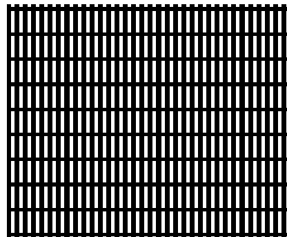
Nr. 4057 mm Lochweite b x h 0,6 x 4,0 Teilung horizontal 1,6 Teilung vertikal 4,8 Durchlass 31 %
