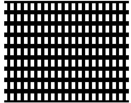
Nr. 1419 mm Lochweite b x h 1,5 x 3,0 Teilung horizontal 3,0 Teilung vertikal 5,0 Durchlass 30 %
