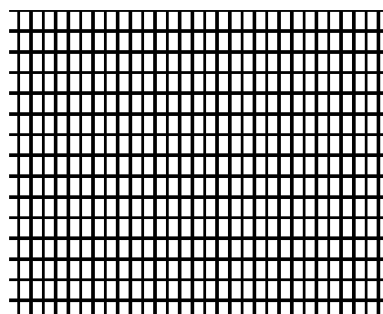
Nr. 4310 mm Lochweite b x h 1,2 x 2,4 Teilung horizontal 1,8 Teilung vertikal 3,0 Durchlass 53,5 %
