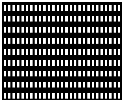
Nr. 4068 mm Lochweite b x h 1,0 x 2,5 Teilung horizontal 2,0 Teilung vertikal 5,0 Durchlass 25 %
