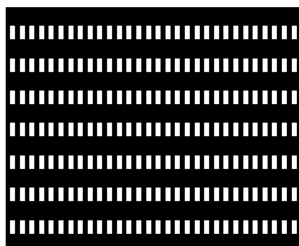
Nr. 4130 mm Lochweite b x h 0,9 x 2,5 Teilung horizontal 1,8 Teilung vertikal 6,0 Durchlass 21 %
