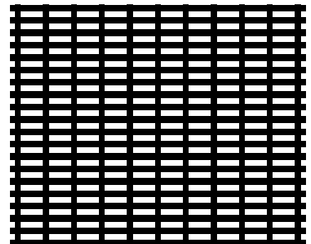
Nr. 4063 mm Lochweite b x h 4,0 x 1,0 Teilung horizontal 5,2 Teilung vertikal 2,3 Durchlass 35 %
