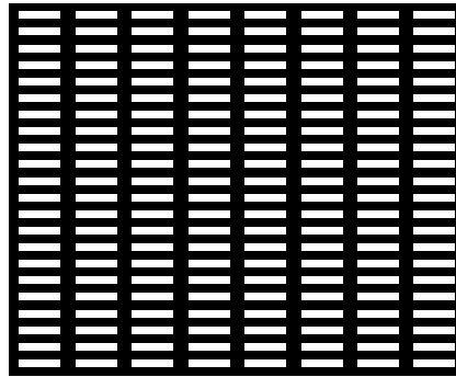
Nr. 4000 mm Lochweite b x h 5,0 x 0,8 Teilung horizontal 6,8 Teilung vertikal 2,0 Durchlass 31 %
