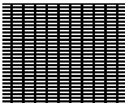
Nr. 4132 mm Lochweite b x h 4,0 x 0,6 Teilung horizontal 5,22 Teilung vertikal 1,6 Durchlass 29 %
