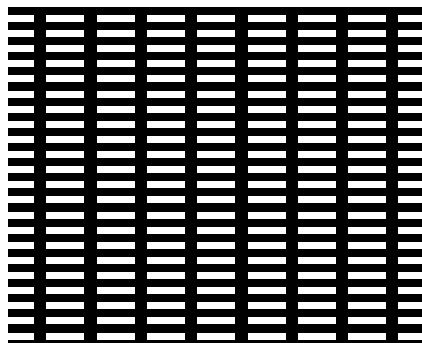
Nr. 4056 mm Lochweite b x h 5,0 x 0,8 Teilung horizontal 6,65 Teilung vertikal 2,0 Durchlass 31 %
