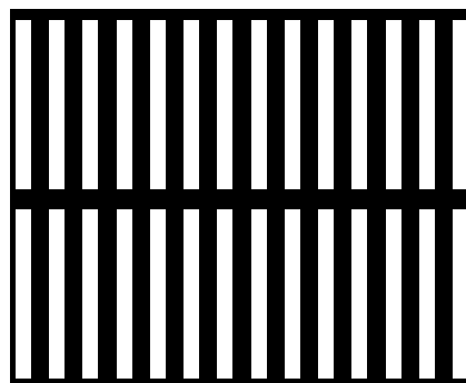
Nr. 4072 mm Lochweite b x h 1,8 x 20 Teilung horizontal 4,0 Teilung vertikal 22,5 Durchlass 40 %
