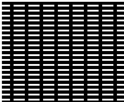
Nr. 4069 mm Lochweite b x h 5,0 x 0,75 Teilung horizontal 6,6 Teilung vertikal 2,2 Durchlass 25 %
