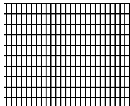
Nr. 4313 mm Lochweite b x h 1,5 x 3,9 Teilung horizontal 2,1 Teilung vertikal 4,5 Durchlass 62 %
