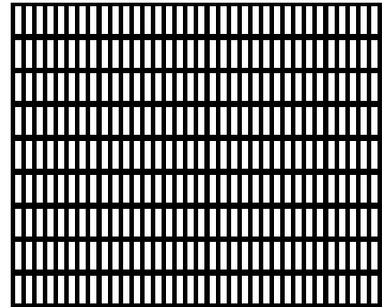
Nr. 4055 mm Lochweite b x h 0,8 x 4,0 Teilung horizontal 1,6 Teilung vertikal 5,0 Durchlass 42 %
