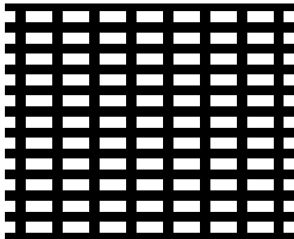
Nr. 1499 mm Lochweite b x h 5,0 x 2,0 Teilung horizontal 7,0 Teilung vertikal 4,0 Durchlass 36 %
