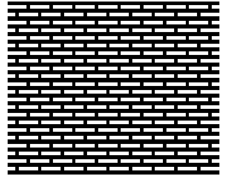
Nr. 4183 mm Lochweite b x h 5,0 x 0,8 Teilung horizontal 5,9 Teilung vertikal 2,0+2,0 Durchlass 34 %
