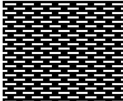
Nr. 1491 mm Lochweite b x h 5,0 x 0,8 Teilung horizontal 8,0 Teilung vertikal 2,0+2,0 Durchlass 25 %
