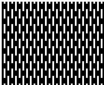
Nr. 4305 mm Lochweite b x h 0,85 x 5,0 Teilung horizontal 2,0+2,0 Teilung vertikal 8,0 Durchlass 26,5 %
