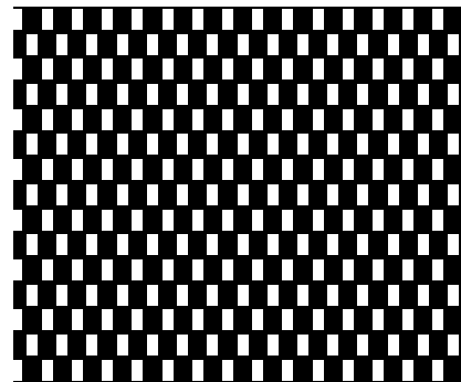
Nr. 4349 mm Lochweite b x h 1,2 x 2,4 Teilung horizontal 1,8+1,8 Teilung vertikal 6,0 Durchlass 26,7 %
