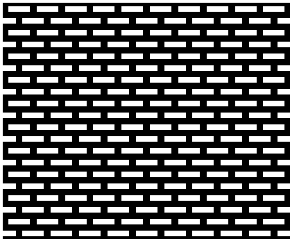
Nr. 1490 mm Lochweite b x h 4,0 x 1,0 Teilung horizontal 5,4 Teilung vertikal 2,25+2,25 Durchlass 33 %
